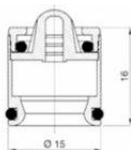
MSCLMT0815001 Limitatore di flusso 8 lt/min
