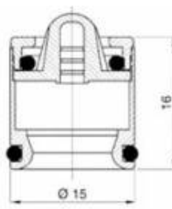
MSCLMT1015023 Limitatore di flusso 10 lt/min
