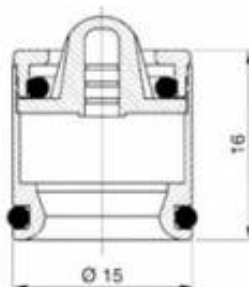
MSCLMT1015023 Limitatore di flusso 10 lt/min
