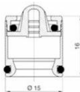
MSCLMT0615018 Limitatore di flusso 6 lt/min
